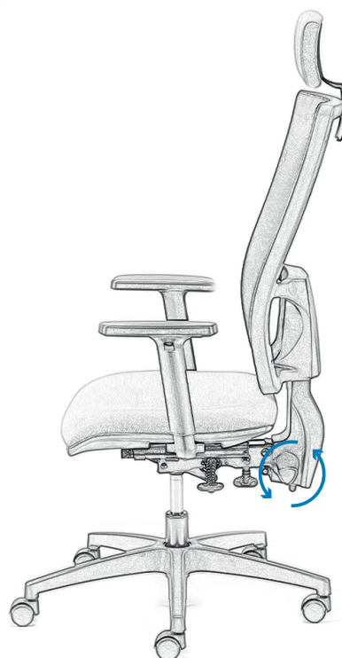
EN Adjusting the height of the backrest by locking the handwheel FR Réglage de la hauteur du dossier par verrouillage du bouton PL Regulacja wysokości oparcia przez blokowanie pokrętle
