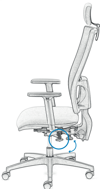
EN Synchronized adjustment of the tilt angle of the backrest and seat by means of the left lever FR Réglage synchronisé de l'angle d'inclinaison du dossier et de l'assise au moyen du levier gauche PL Zsynchronizowana regulacja kąta pochylenia oparcia i siedziska za pomocą lewej dźwigni
